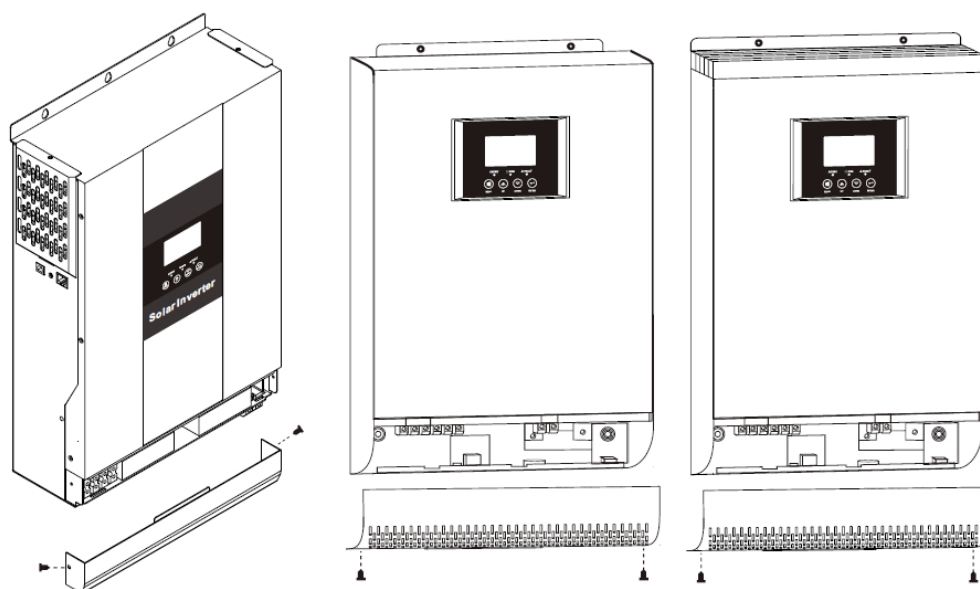
Рисунок 7 Установка защитной крышки
