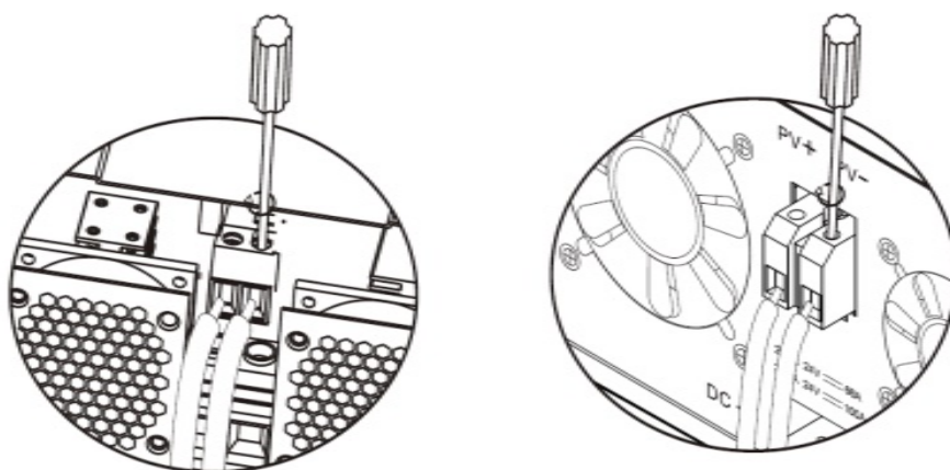
Рисунок 6 Подключение кабеля солнечных панелей
