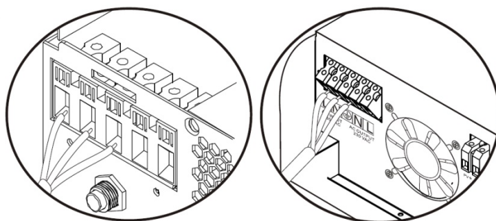
Рисунок 2 Подключение ввода переменного тока
