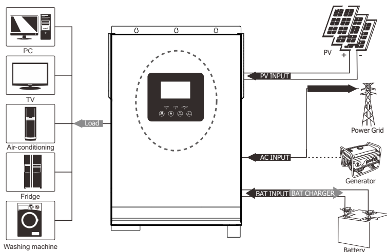
Рисунок 1 Гибридный солнечный инвертор
