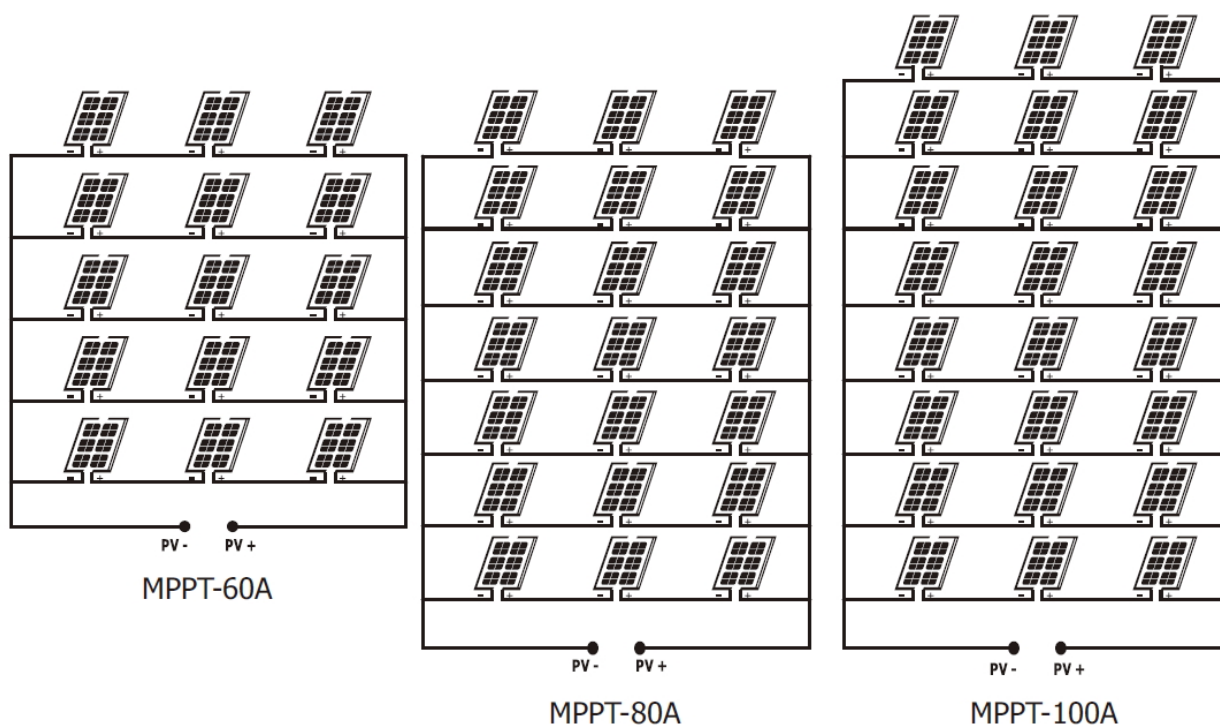
Рисунок 4 Варианты подключения солнечных панелей
